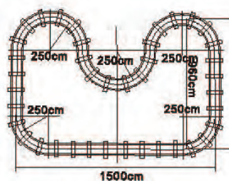
ZZC-8A型追逐车路轨示意图
